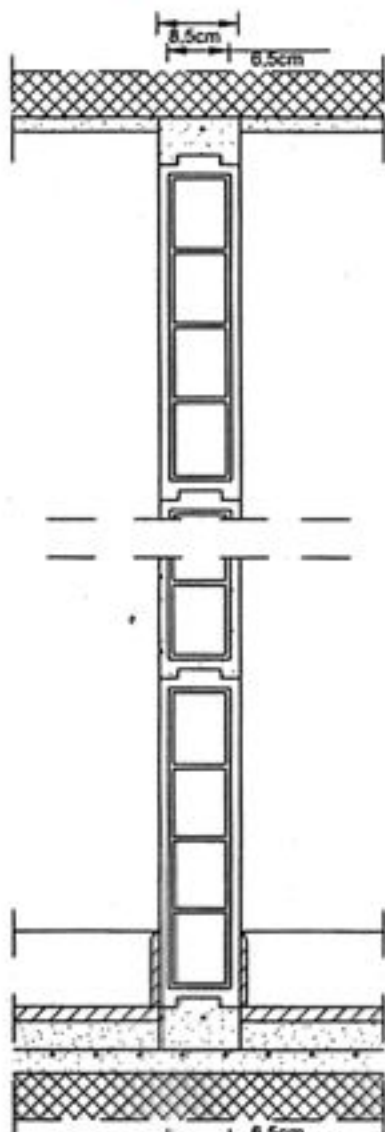
con blocchi in latero-gesso
