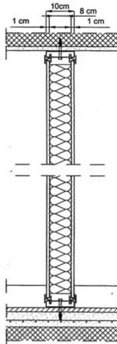
Con guida metallica e pannello sandwich
