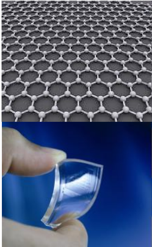
Modello molecolare e porzione di grafene
