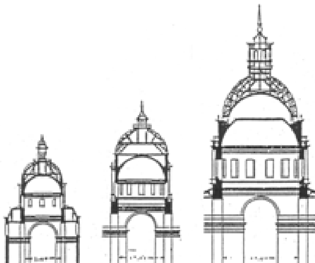
Costruzione francese di cupole rinascimentali
