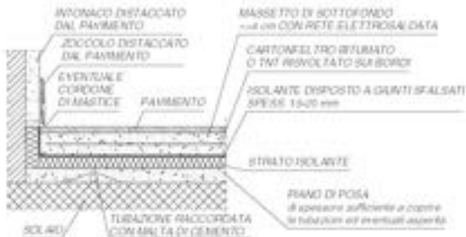
FIG. F.2.3.5 PAVIMENTO GALLEGGIANTE DETTAGLI COSTRUTTIVI
