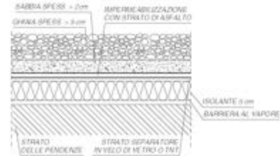
FIG. F.2.5/13 COPERTURE PRATICABILI E NON PRATICABILI
