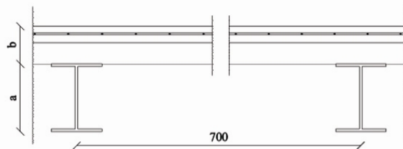
Sezione trasversale (Tipologia 4)
