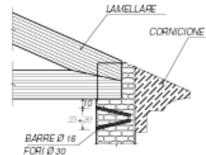
SEZIONE B-B
