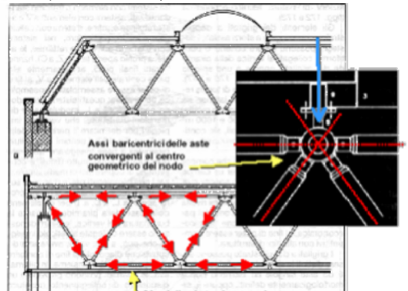
Elementi reticolari
