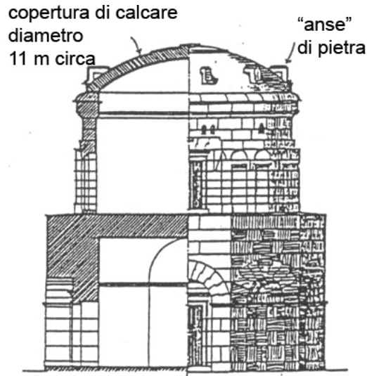
Mausoleo di Teodorico, Ravenna (530) – sezione dell’ opera monolitica di calcare istriano.
