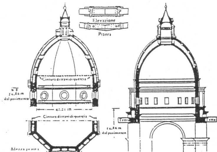
Costruzione di cupole del Rinascimento italiano
