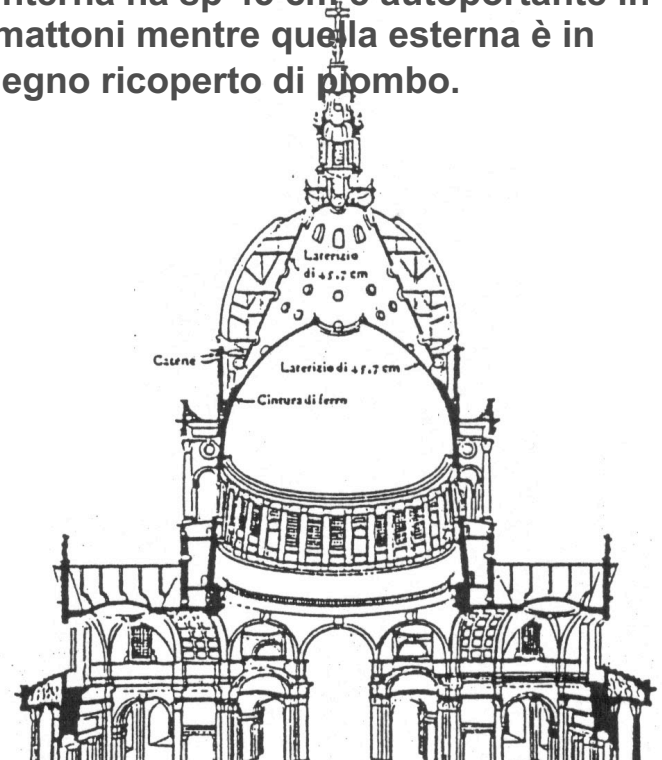
La Cattedrale di San Paolo, Londra 1685-1710
