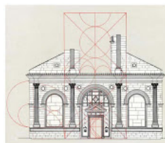
Traccati proporzionali del Tempio Malatestiano, Luca Battista Alberti
