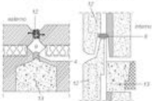
GIUNTO DI PANNELLI MULTISTRATI
