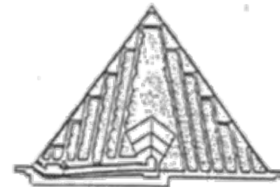
Sezione nord-sud della piramide di Sahure, Abusir Egitto
