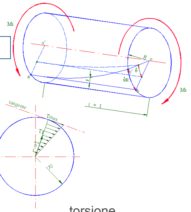
torsione
