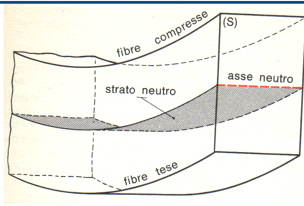
flessione
