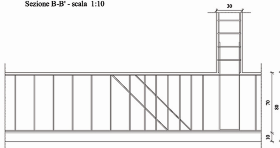
Armadura tipica per trave rovescia - scala 1:20
