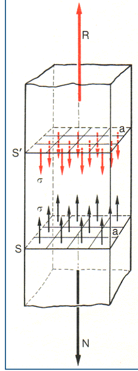
tensione normale
