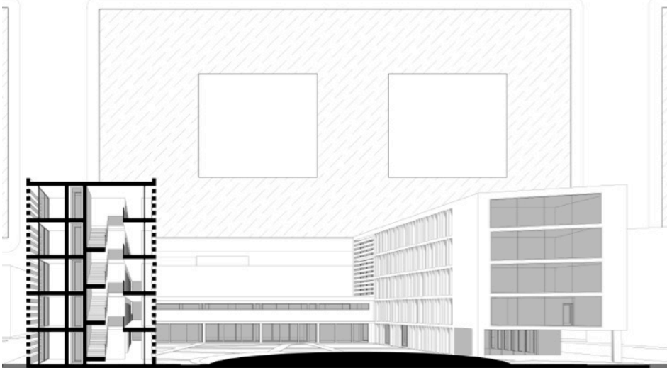
SEZIONE PROSPETTICA B-B, SCALA 1:100
