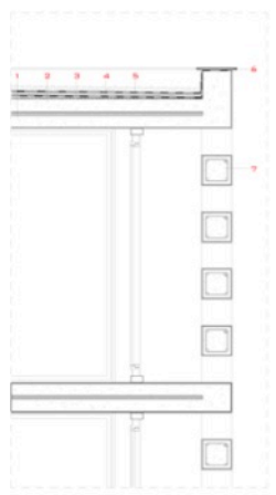
DETTAGLIO COSTRUTTIVO_SCALA 1:20
