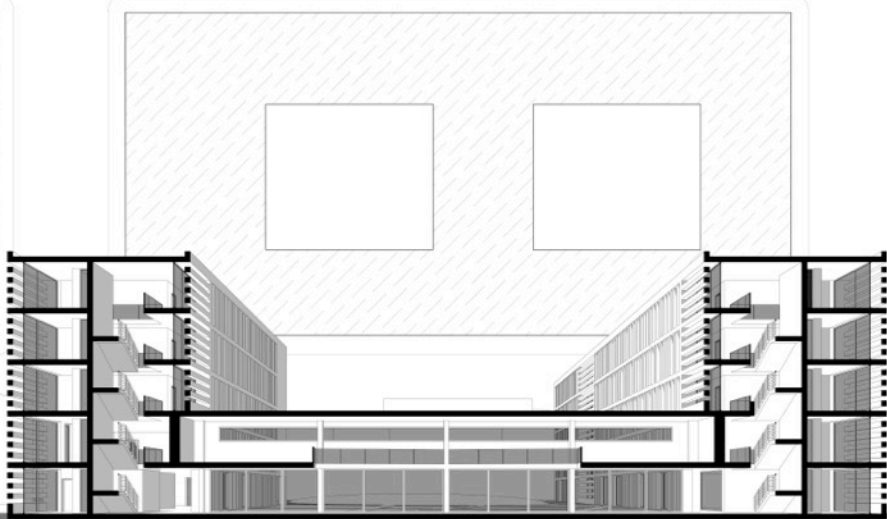
SEZIONE PROSPETTICA A-A, SCALA 1:100
