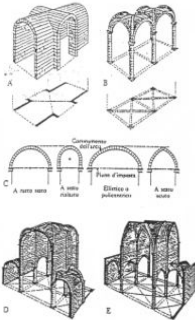
Schemi di costruzioni a volta
